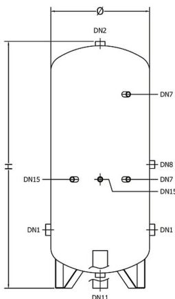
SC/E 750 - 2000
