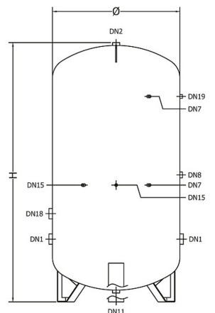
SC/E 3000 - 5000
